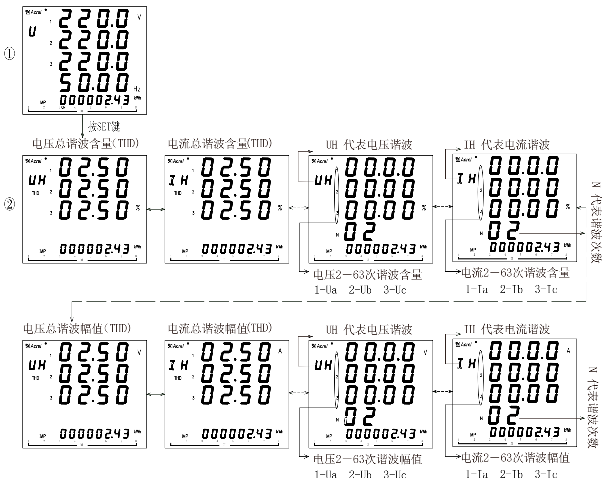
相电压显示界面
