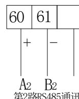
第2路RS485通讯
