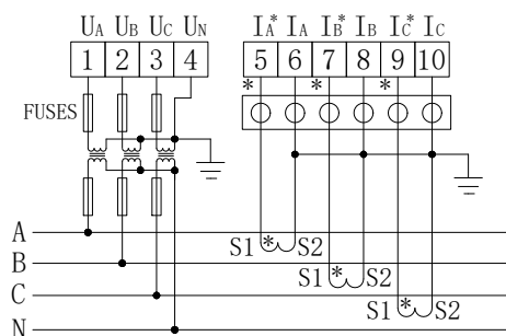
三相四线3PT、3CT
