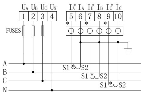
三相四线3CT
