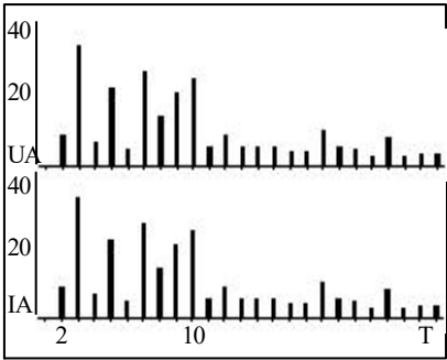
谐波棒图
