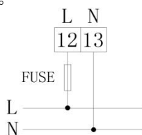
辅助电源
