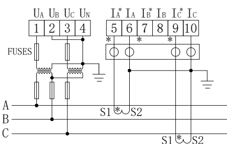
三相三线2PT、2CT
