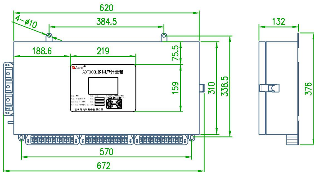
图 3 ADF300L-III 尺寸
