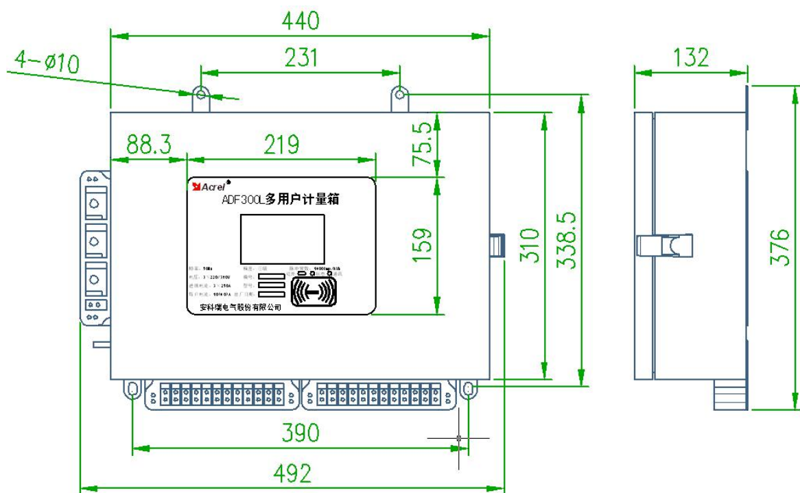
图 2 ADF300L-II 尺寸
