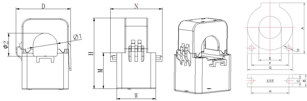
图 3 配套互感器尺寸图
