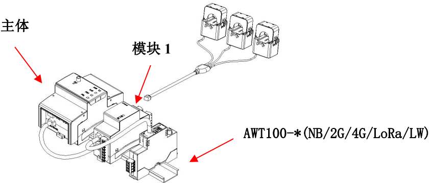
图 4 导轨式安装
