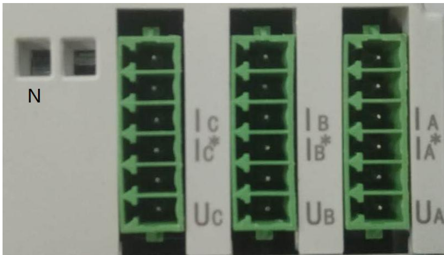
AEW100-D15、AEW100-D15W、AEW100-D20W、AEW100-D36W 端子图
