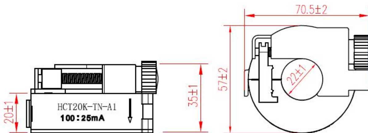
图 5 配套互感器 HCT20K-TN 尺寸图
