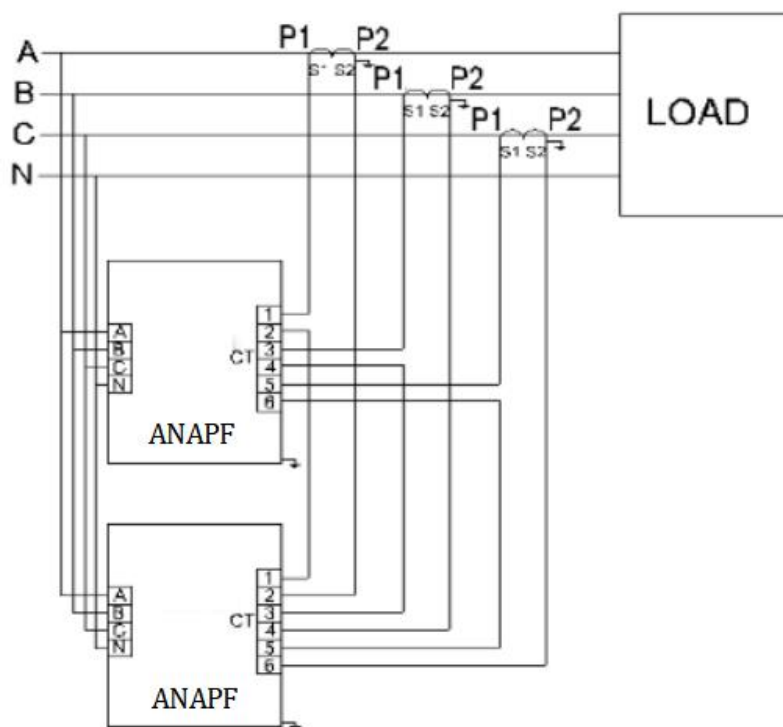
图 4-2 电流互感器安装位置及多 ANAPF 并联电流互感器接线示意图
