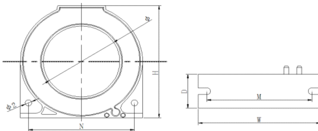
互感器部分
