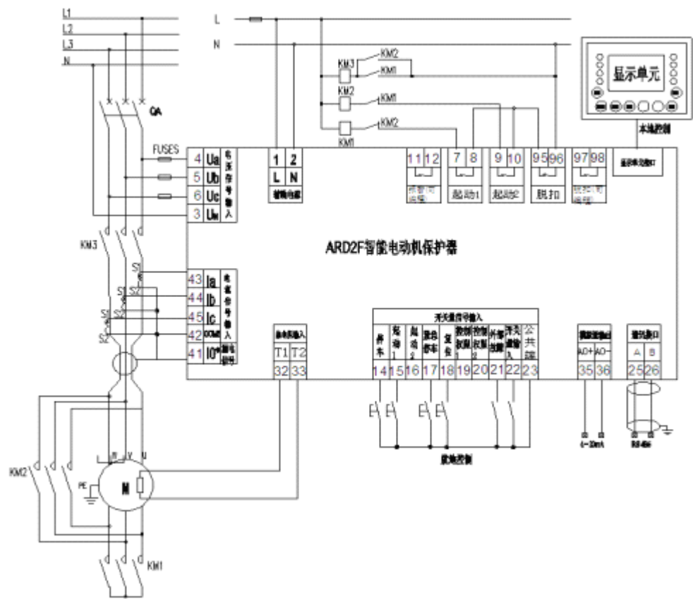
ARD2F 电动机保护器 Y-△起动模式接线图（适用于 1.6、6.3、25、100、250、800A 电流规格）：
