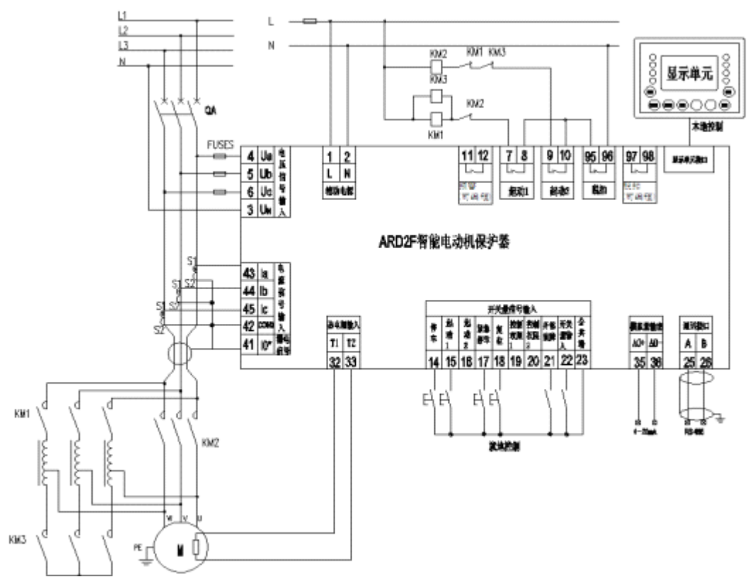
ARD2F 电动机保护器自耦降压起动模式接线图（适用于 1.6、6.3、25、100、250、800A 电流规格）：
