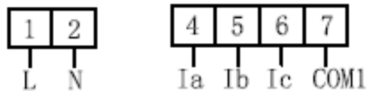
辅助电源
