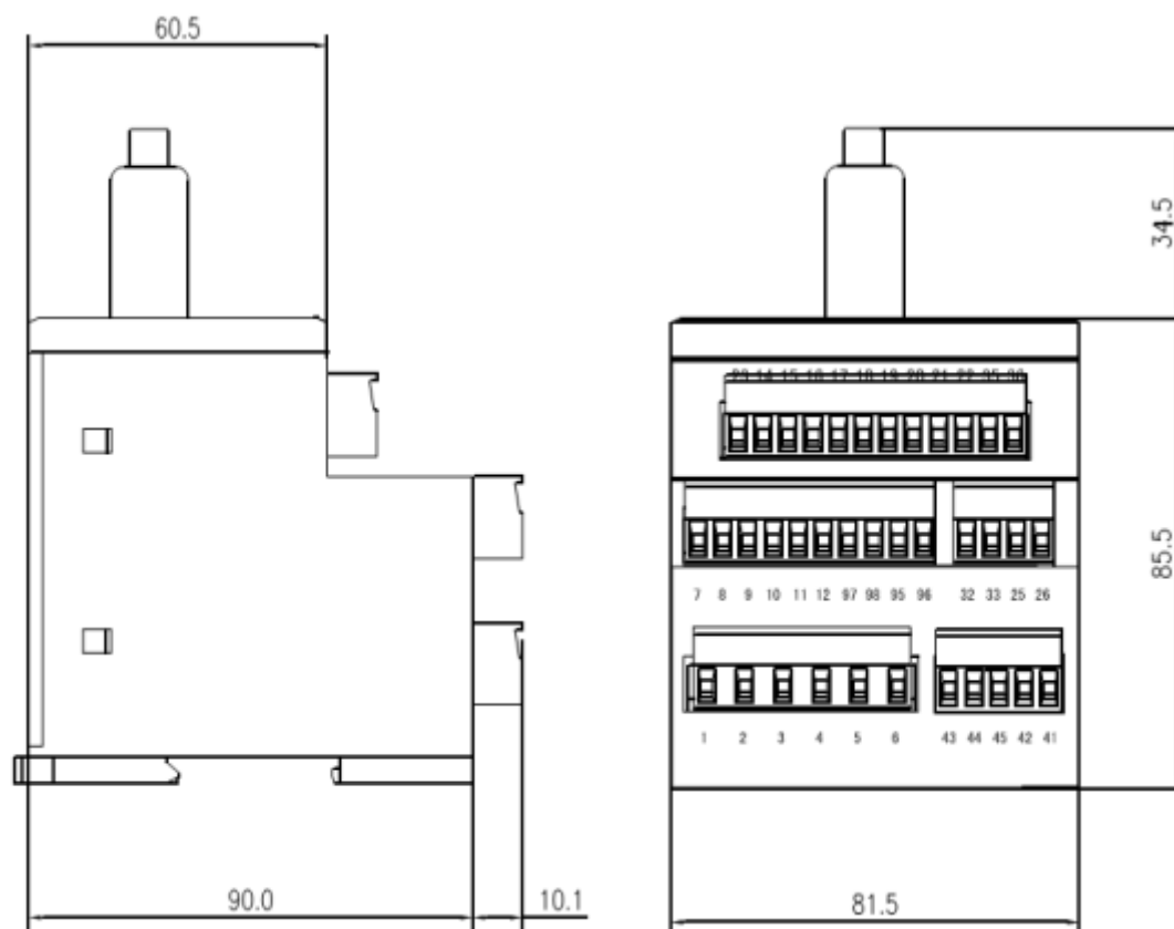
主视图
