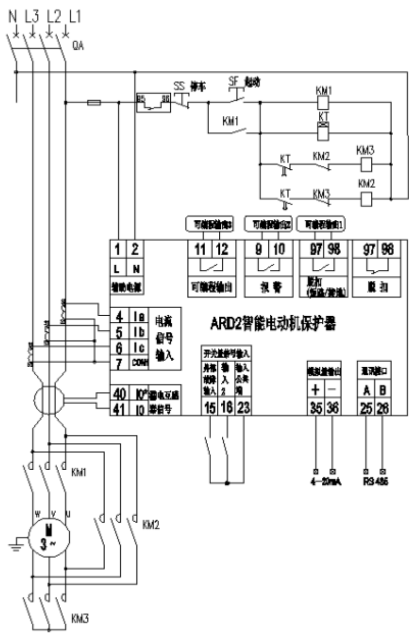
ARD2 电动机保护器 Y-△起动模式接线图 (适用于 1.6、6.3、25、100、250、800A 电流规格)
