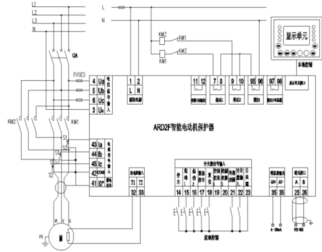
ARD2F 电动机保护器正反转起动模式接线图（适用于 1.6、6.3、25、100、250、800A 电流规格）：
