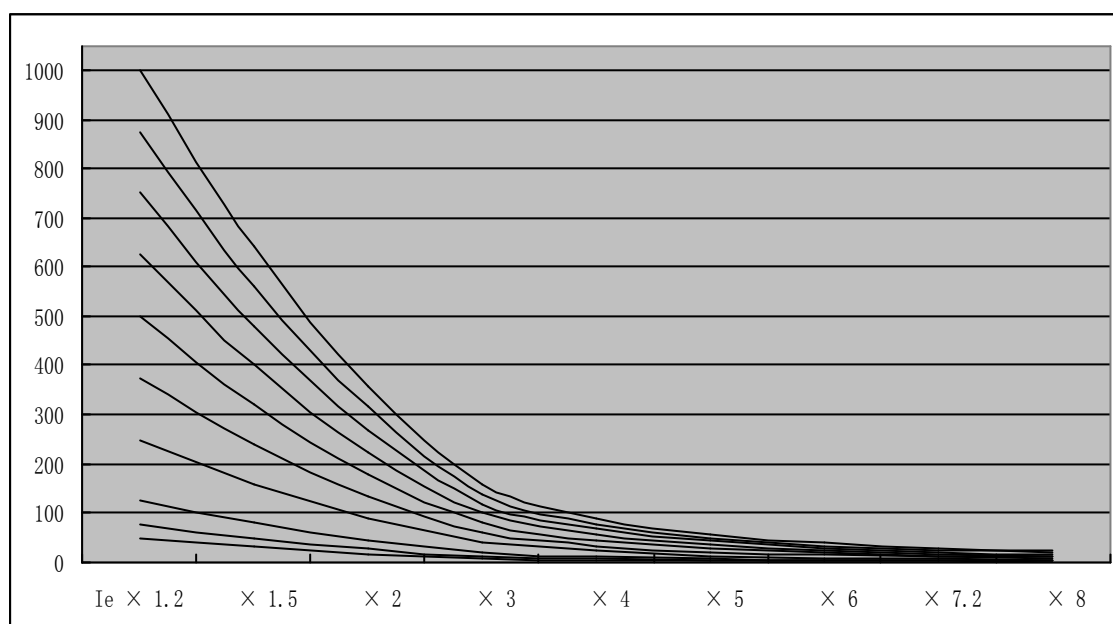
过载特征曲线图 (K 曲线图)
