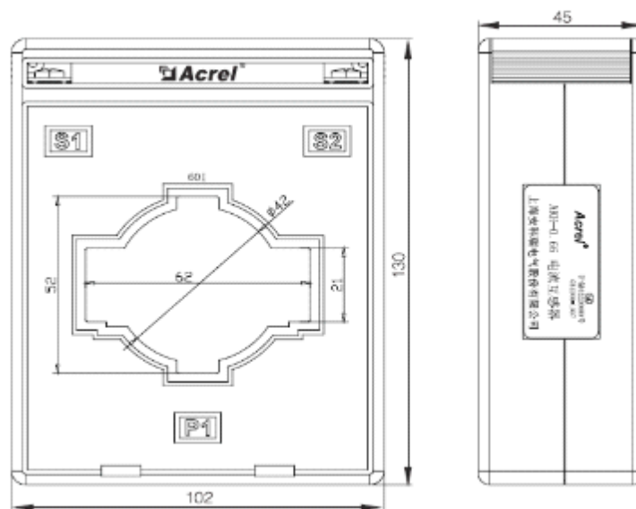
互感器部分（保护器电流规格为 800A 时所配电流互感器）
