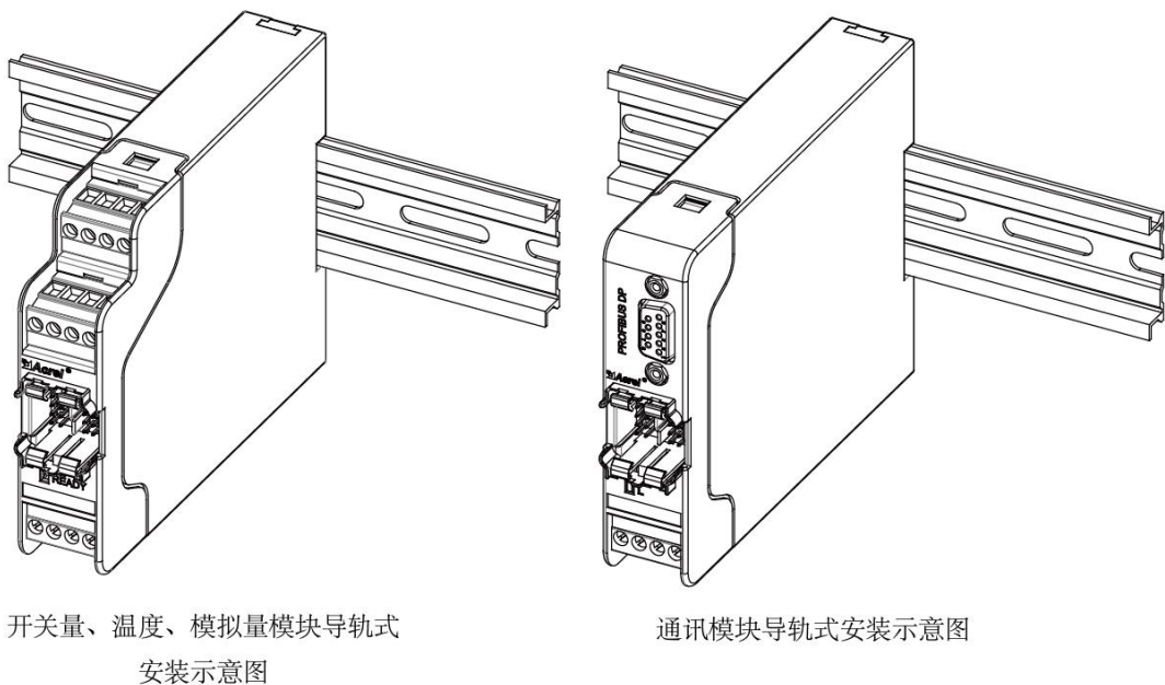
图 14 导轨安装
