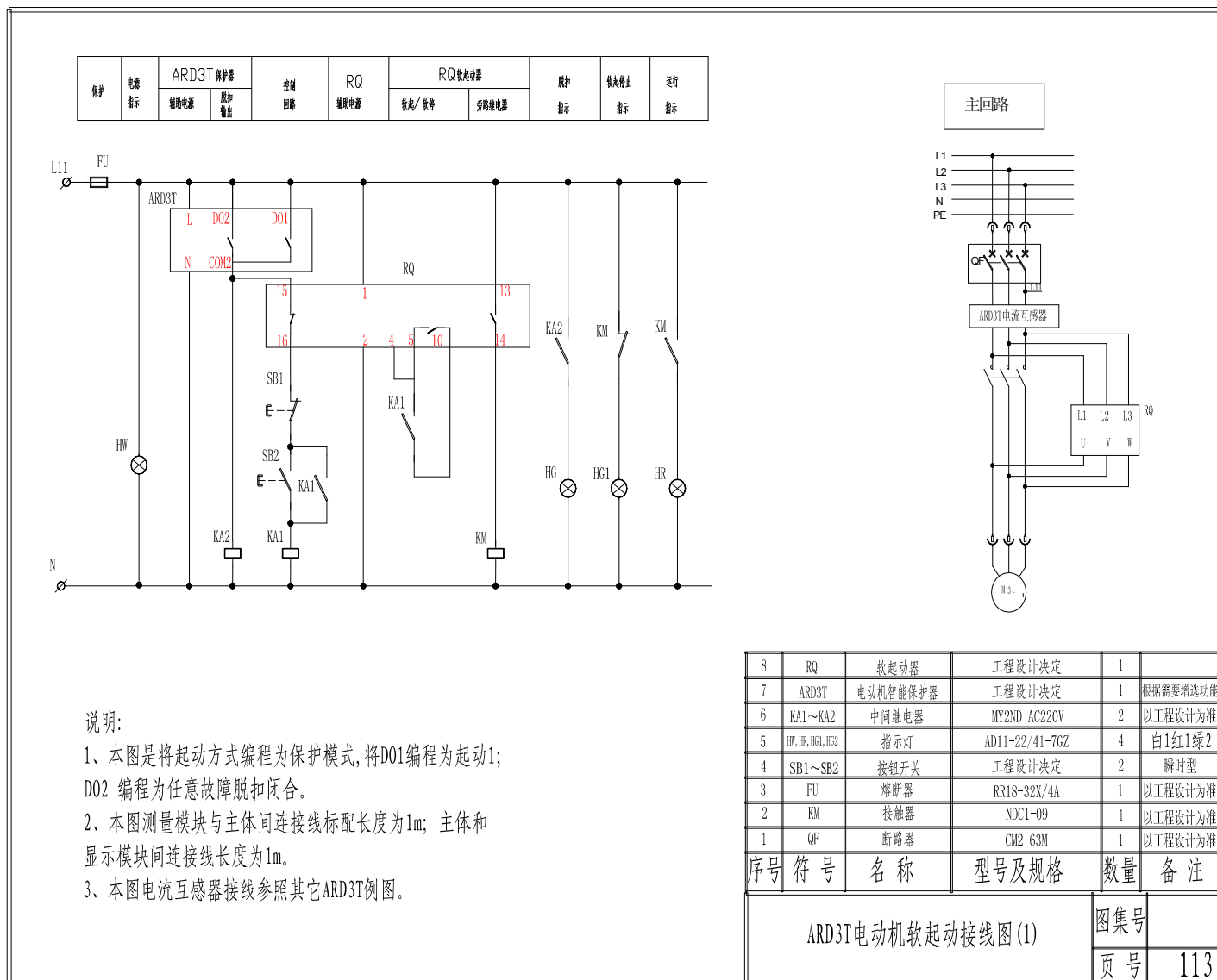
9.10 ARD3T 软起动接线图 (1)
