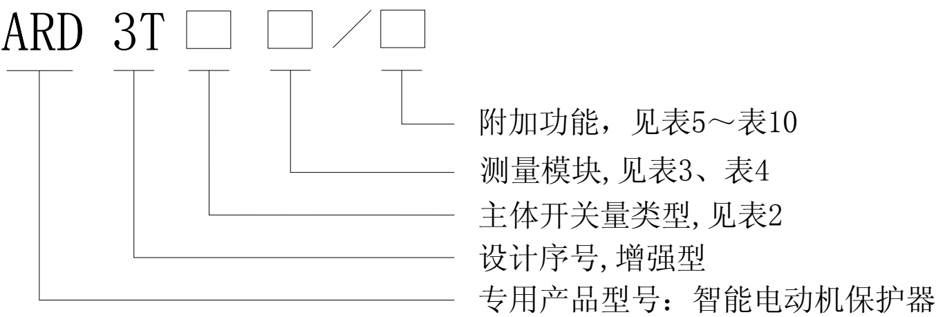
图 3 选型说明
