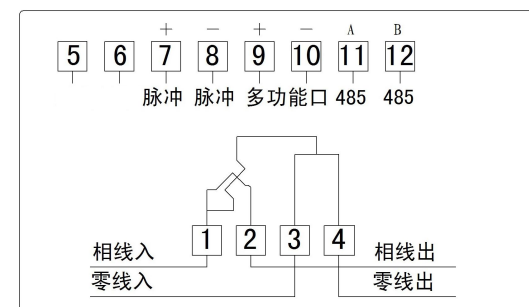
图二（1）直接接入式
