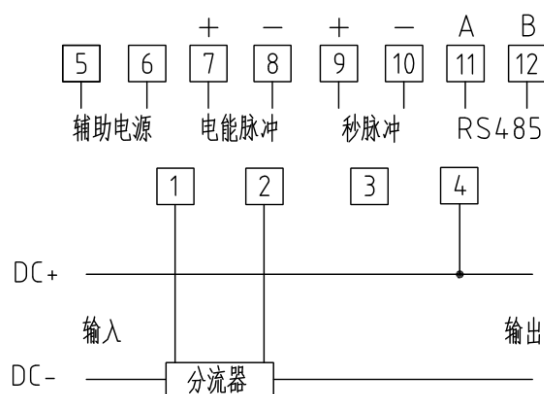
图 3 分流器接线图
