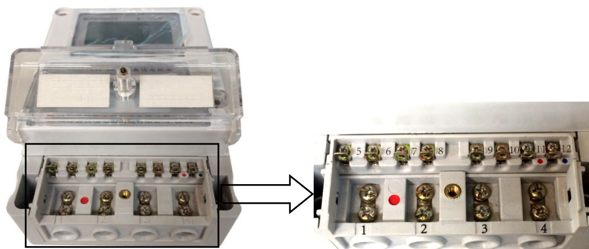
图 2 端子接线图
