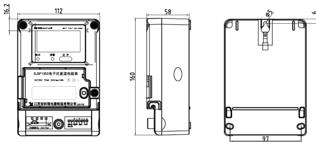
图 1 外观尺寸
