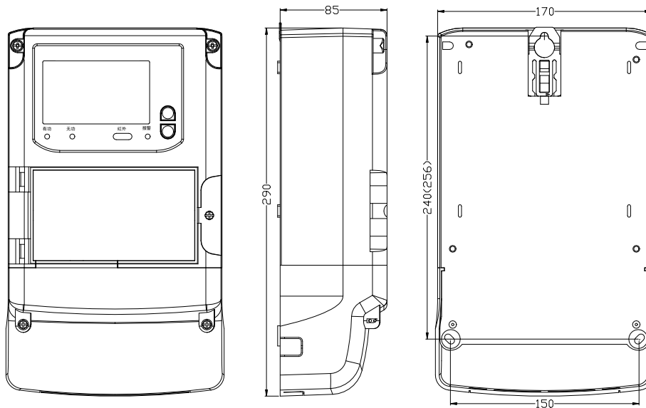
外形示意图
