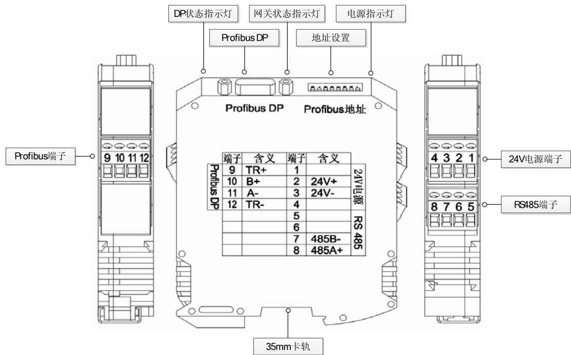
图 4：接线图
