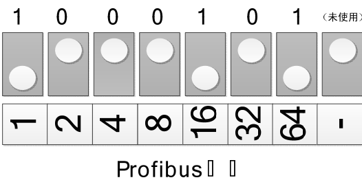
图 5：Profibus 地址设置示例（设置为 81）
